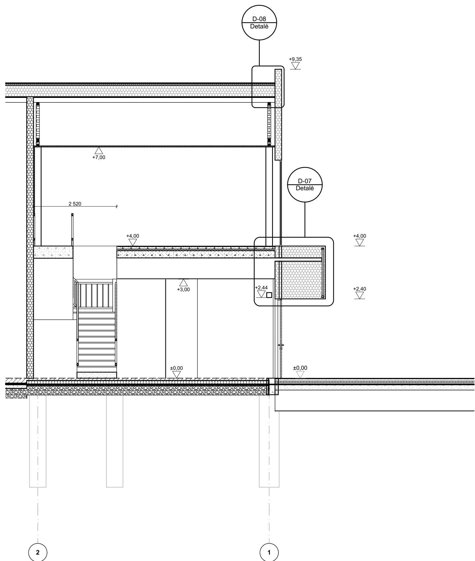
A-A Pjuvis 1:70
