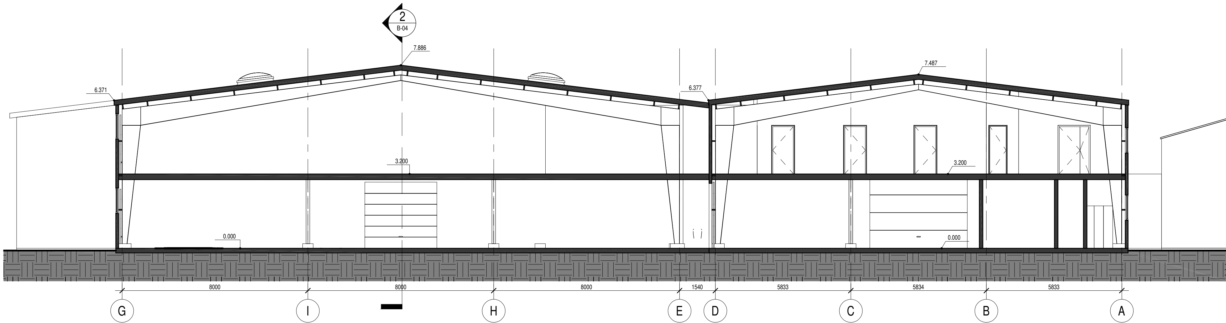
Pjūvis 1-1 1 : 100
