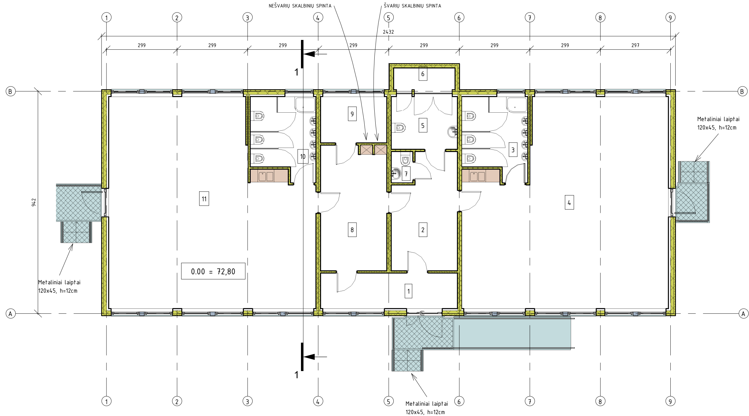
PLANAS 1 : 100
