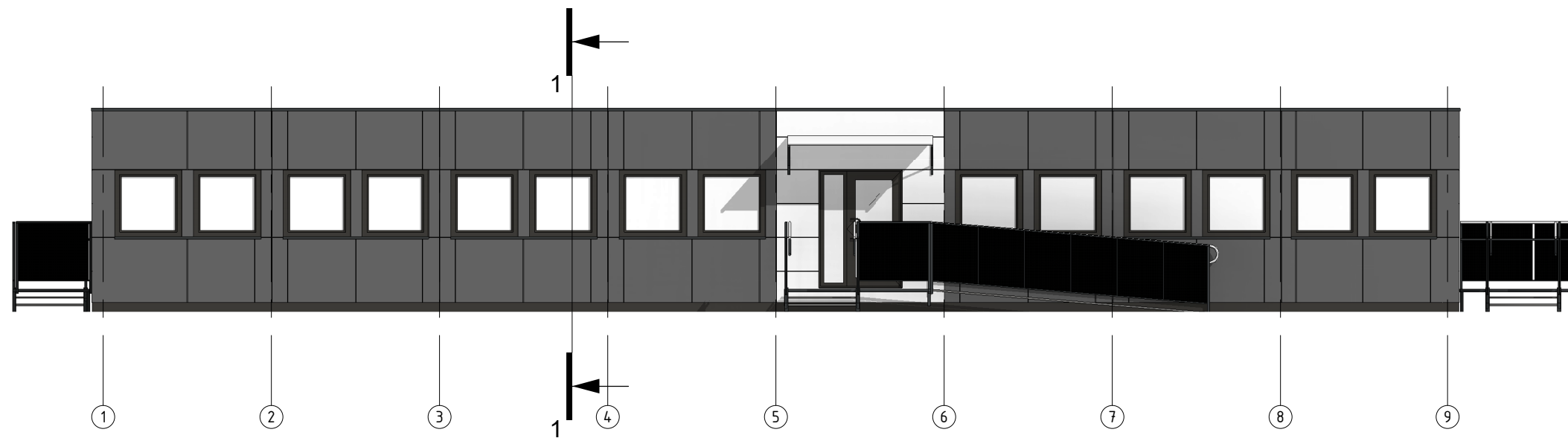
FASADAS 1-9 1 : 100
