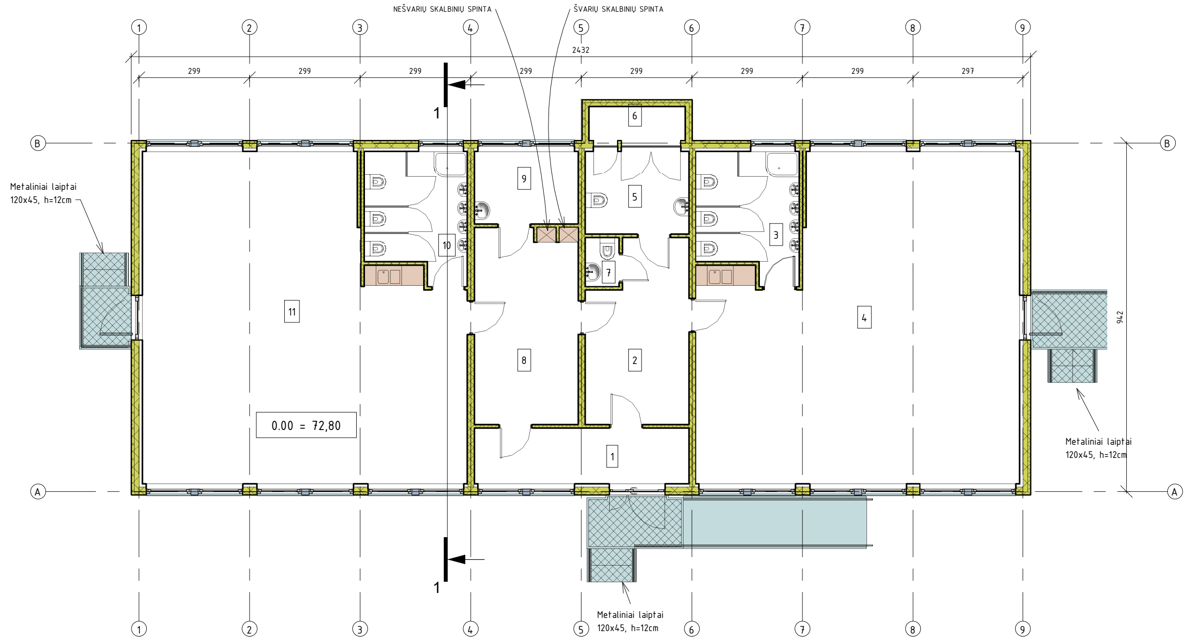
PLANAS 1 : 100
