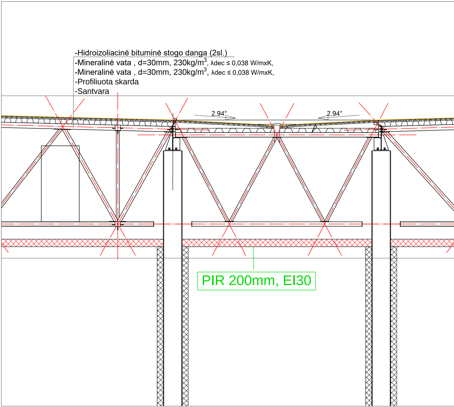
FRAGMENTAS A-A M 1:50
