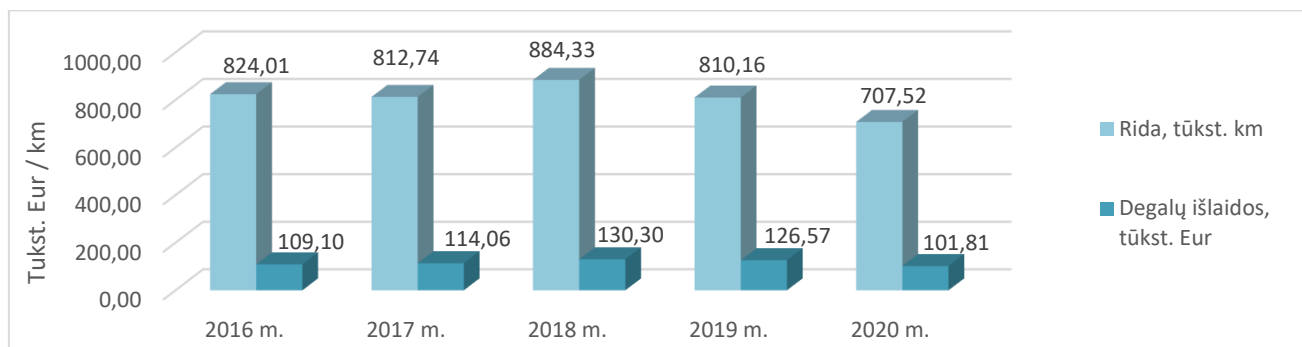
2 pav. Ridos ir degalų išlaidų kaita 2016–2020 m.
