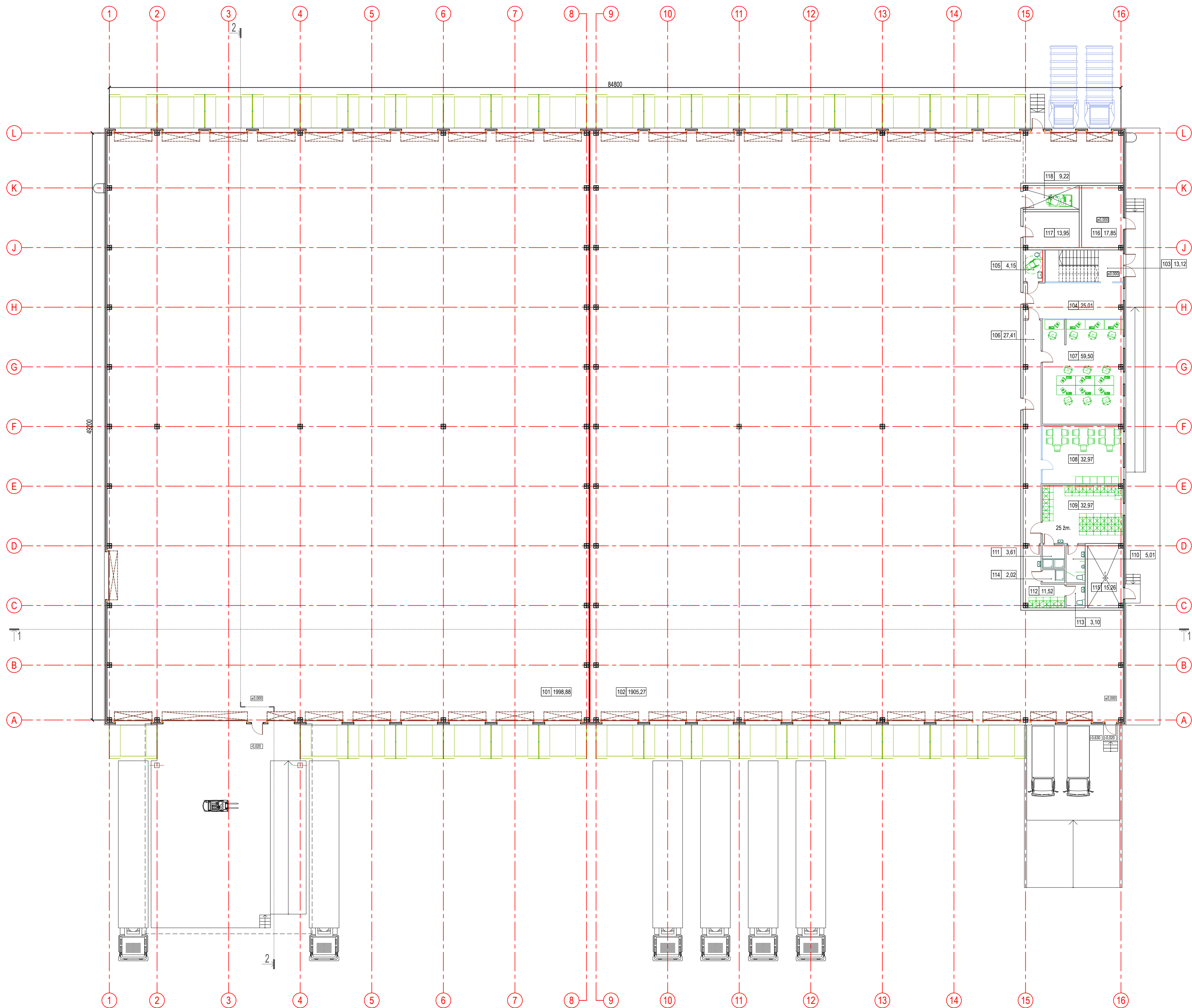
PIRMO AUKŠTO PLANO SCHEMA
