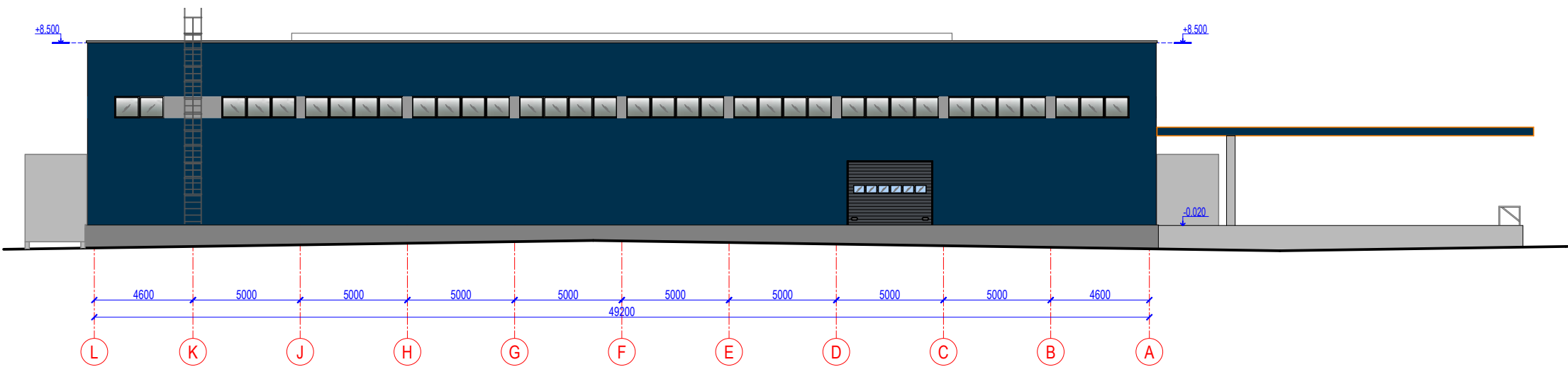
FASADAS "L-A"
