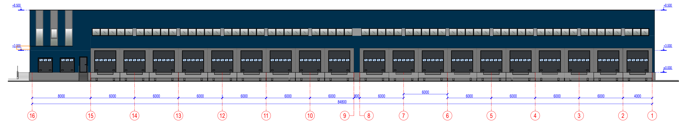
FASADAS "16-1"
