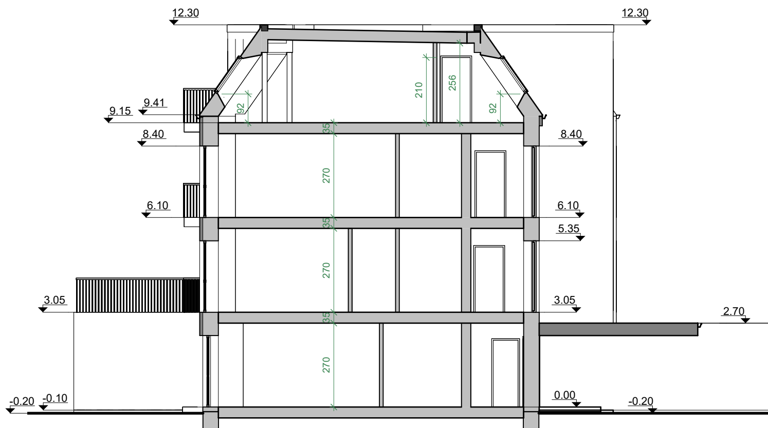
Pjūvis 2-2 1 : 125
