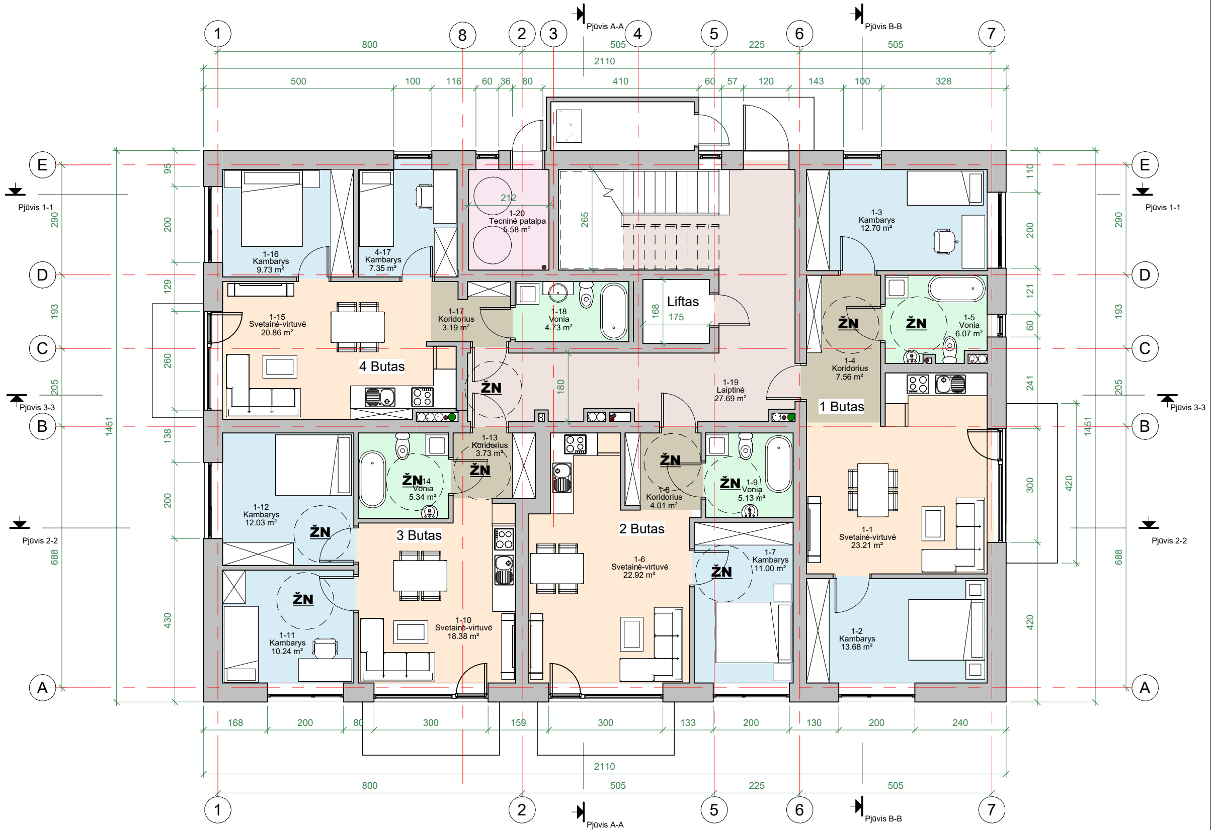
1-Pirmo aukšto planas su baldais 1 : 100
