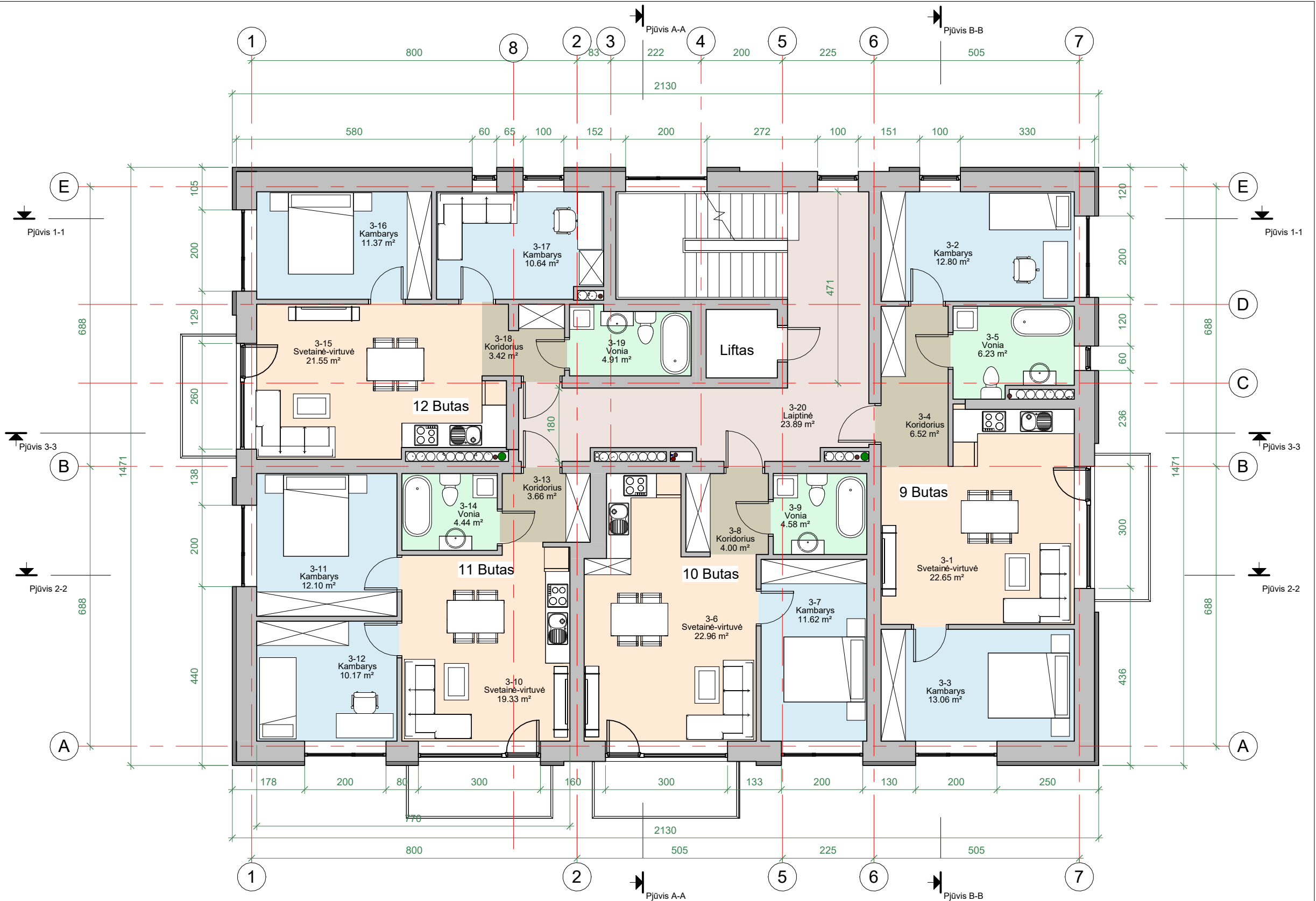
5-Trečio aukšto planas su baldais 1 : 100
