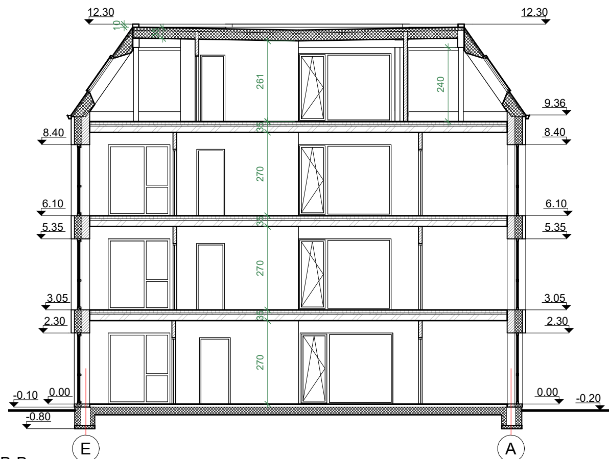
Pjūvis B-B 1 : 125
