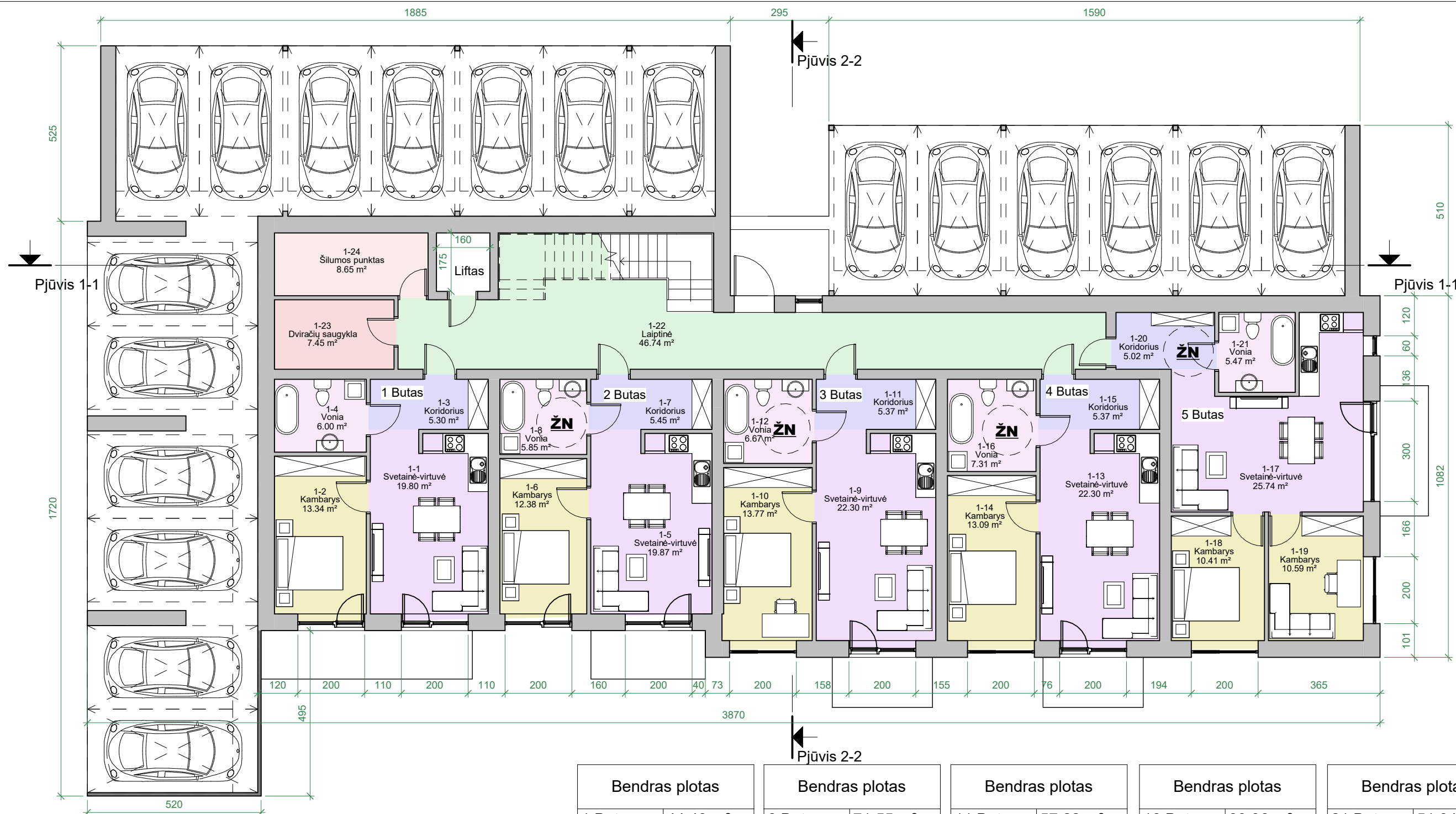
01 Pirmo aukšto planas su baldais 1 : 125
