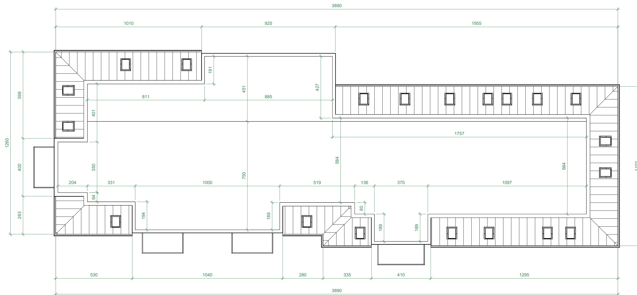
09 Stogo planas 1 : 125
