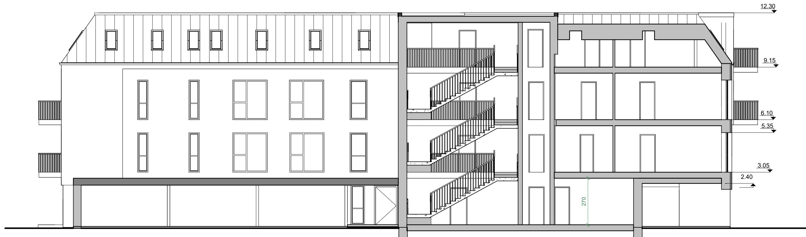
Pjūvis 1-1 1 : 125
