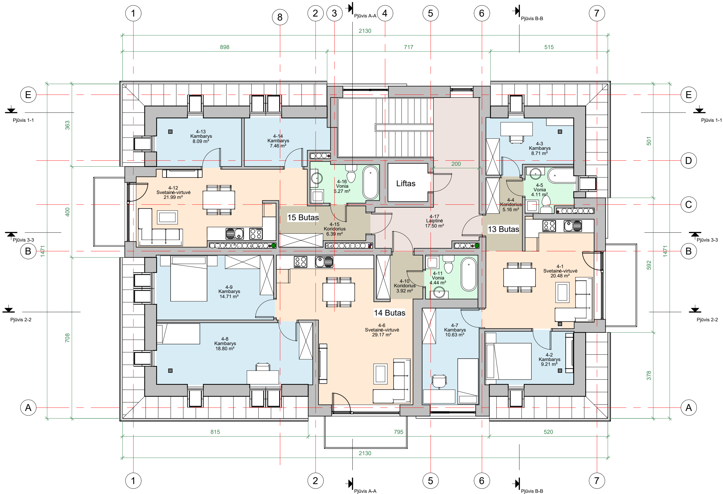
7-Ketvirto aukšto planas su baldais 1 : 100
