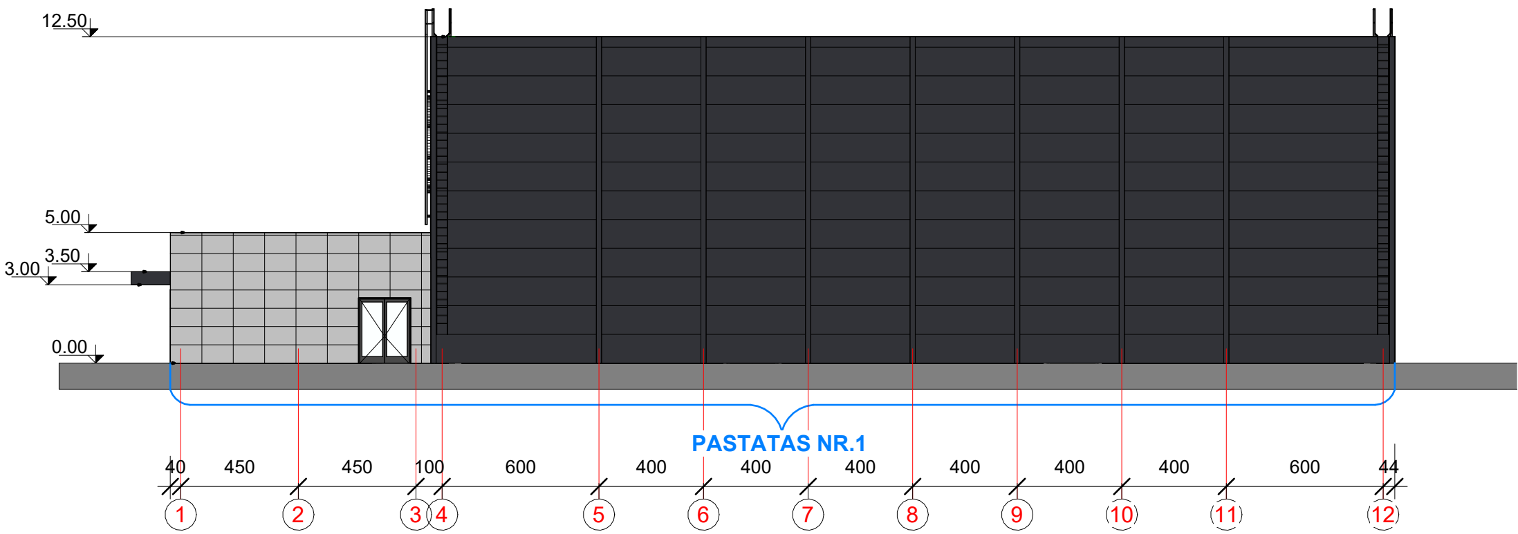
2 Rytinis fasadas 1 : 200
