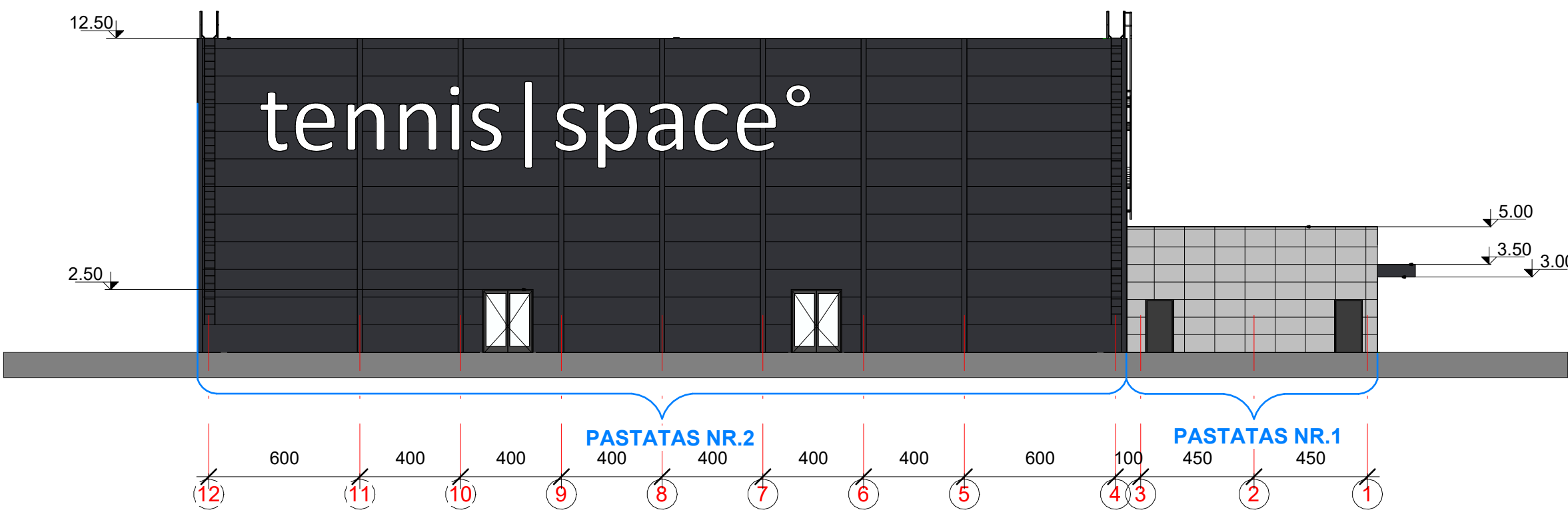
3 Vakarinis fasadas 1 : 200
