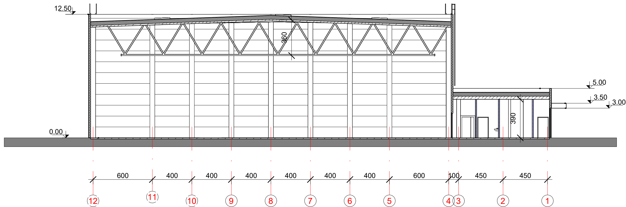
1 Pjūvis A-A 1 : 200
