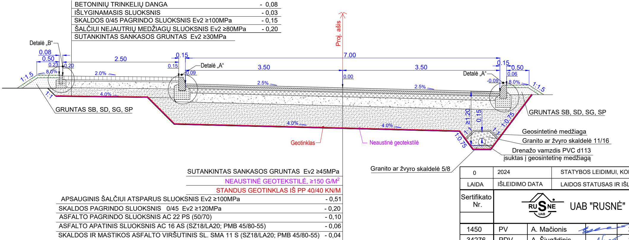
PJŪVIS 2 - 2 M 1:50
