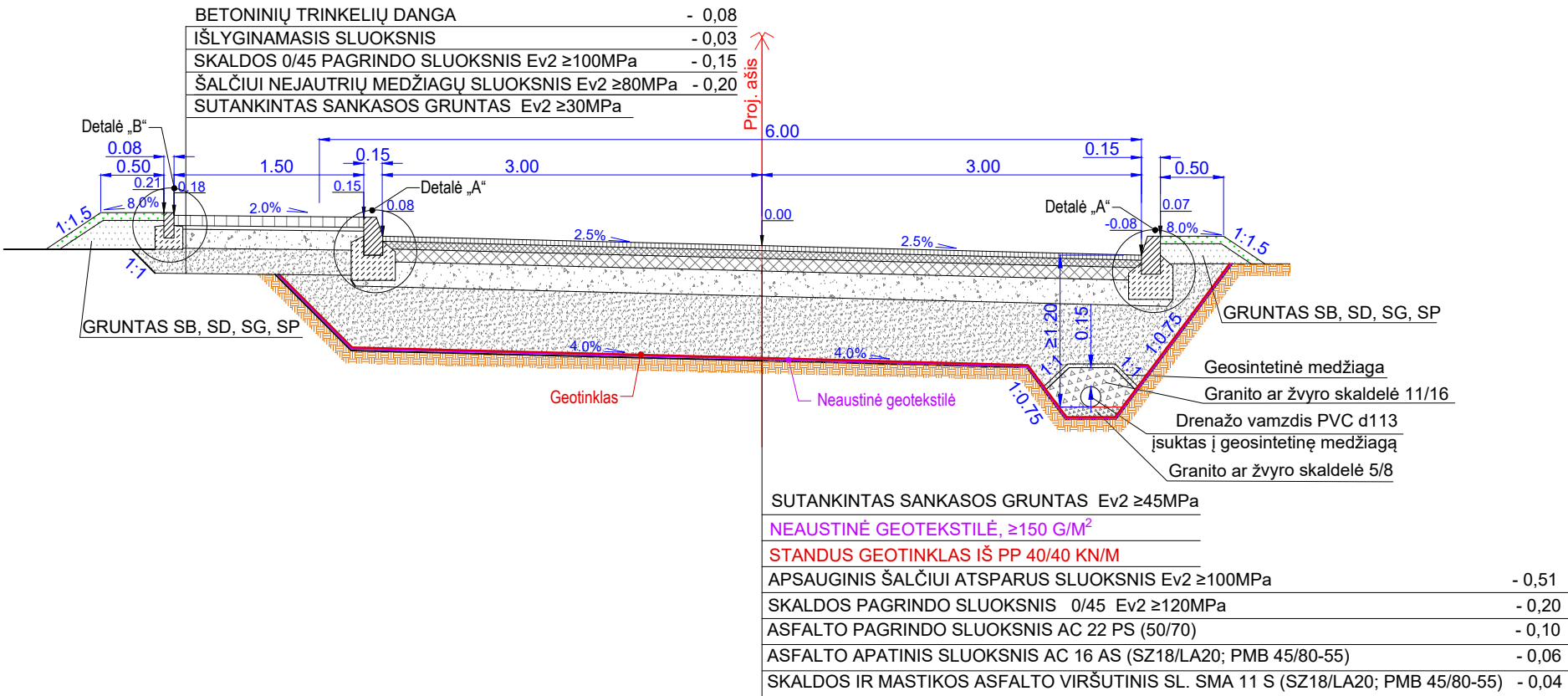
PJŪVIS 1 - 1 M 1:50
