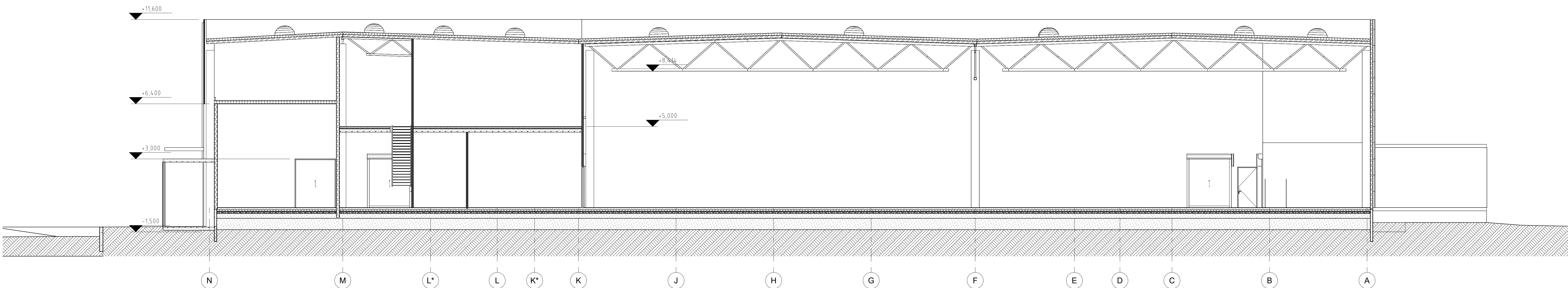
PJŪVIS A-A
