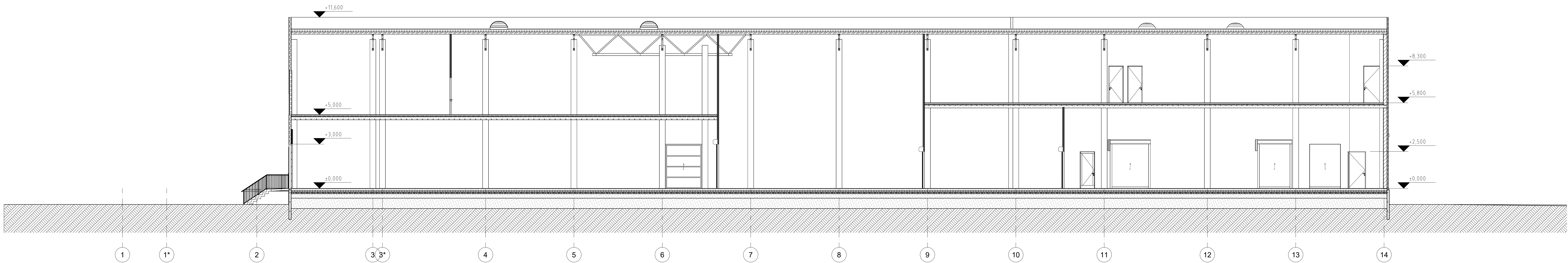
PJŪVIS C-C
