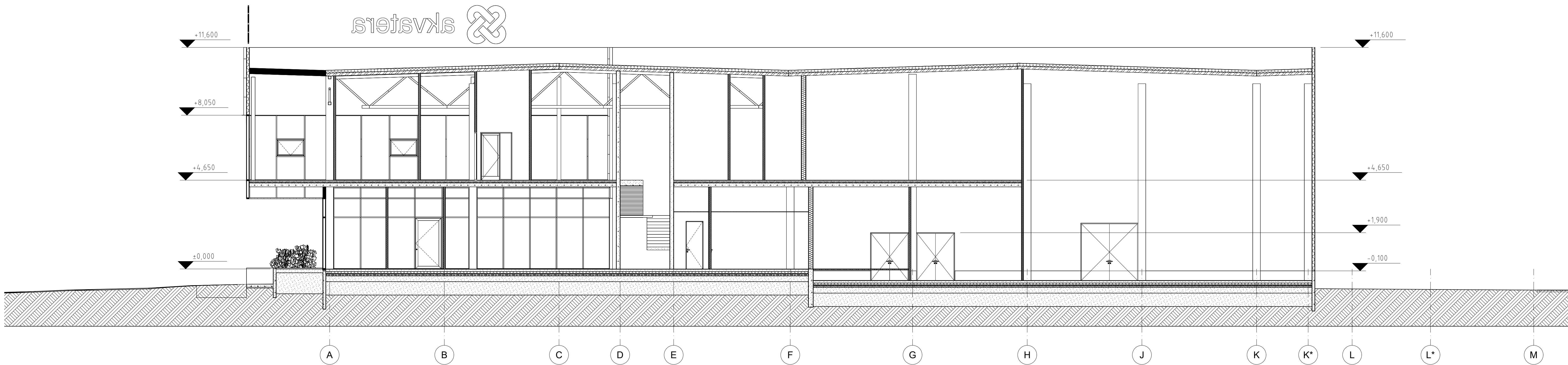
PJŪVIS E-E
