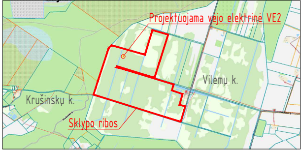
Situacijos schema
