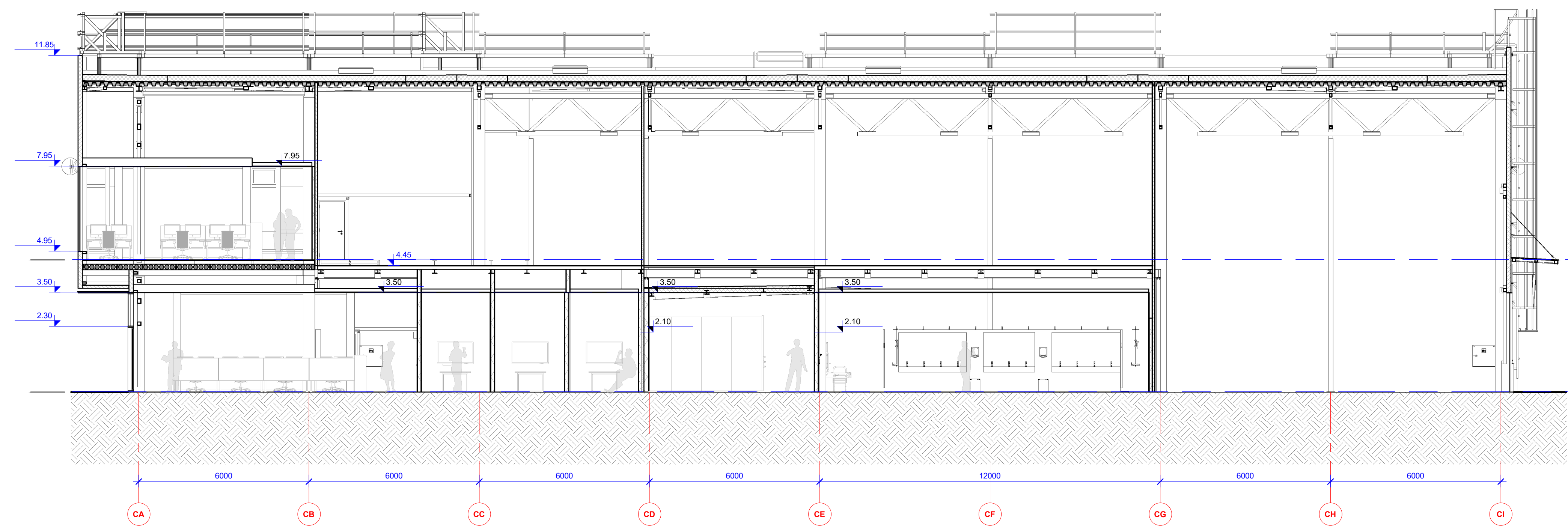
Pjūvis 3-3 MT:100
