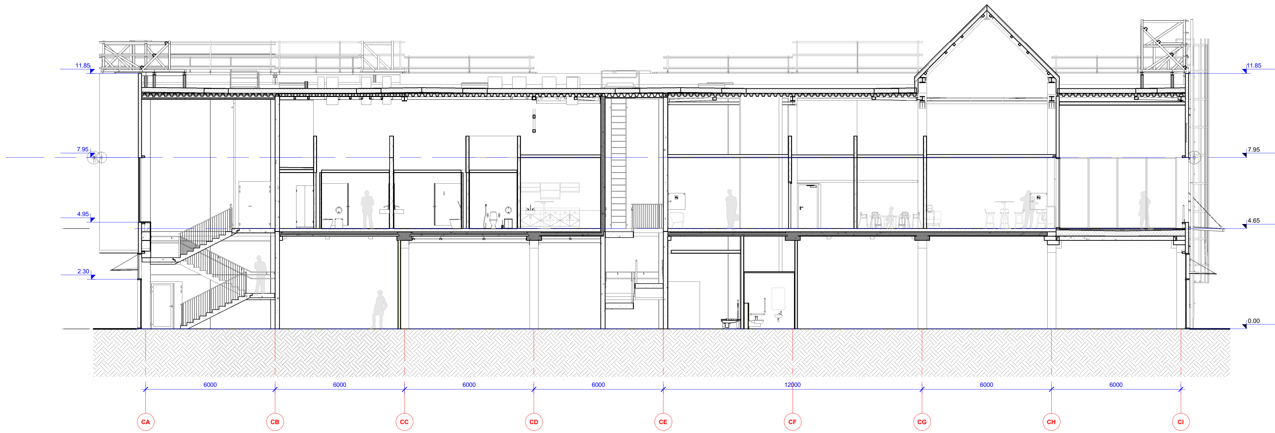
Pjūvis 1-1 MT:100
