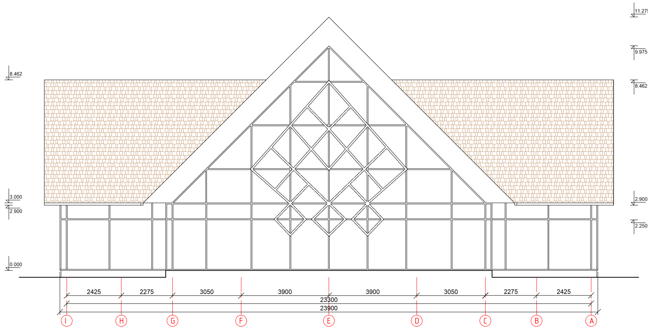
Fasadas I - A M 1:100
