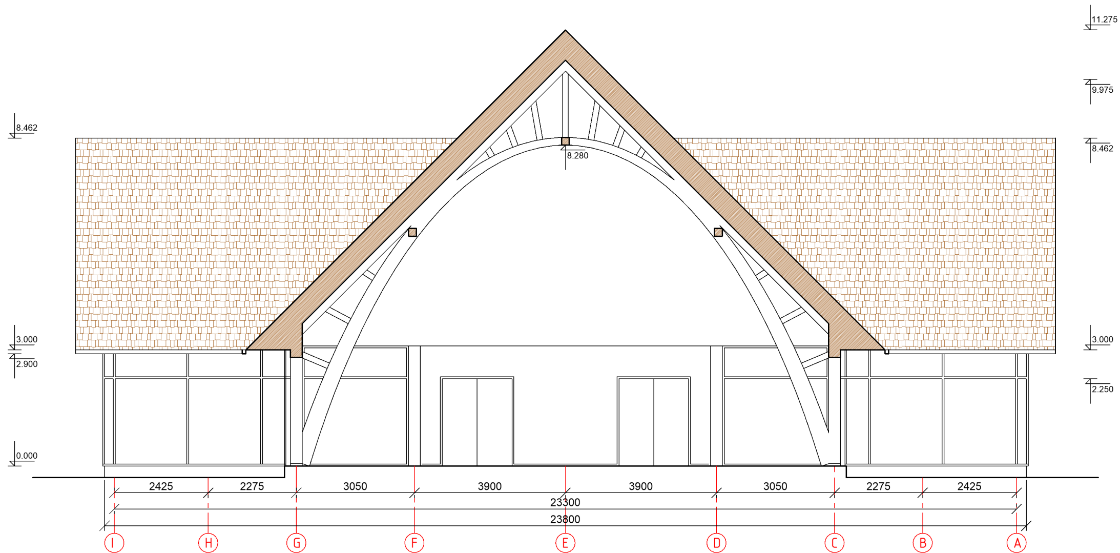
Pjūvis I - A M 1:100
