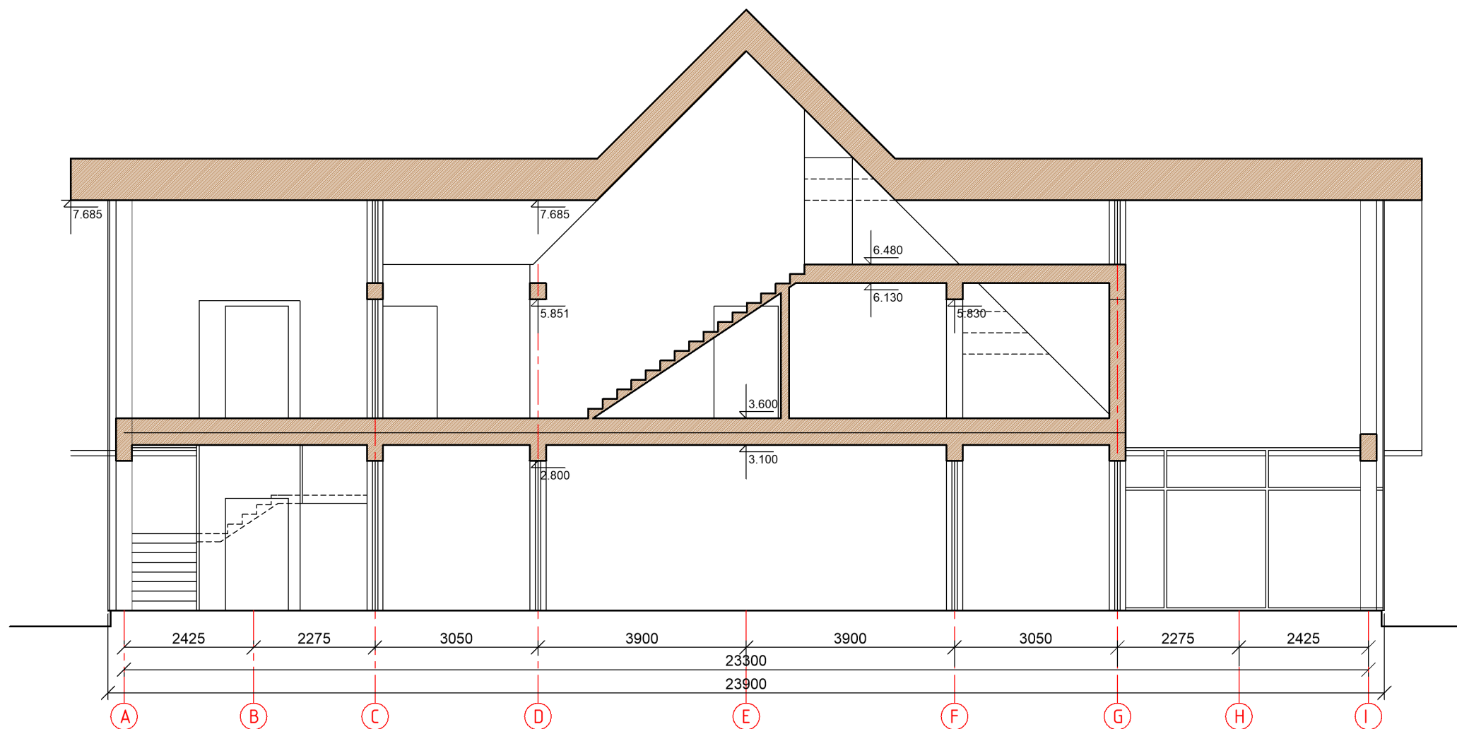
Pjūvis A - I M 1:100
