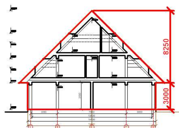
Projektuojamas pastatas
