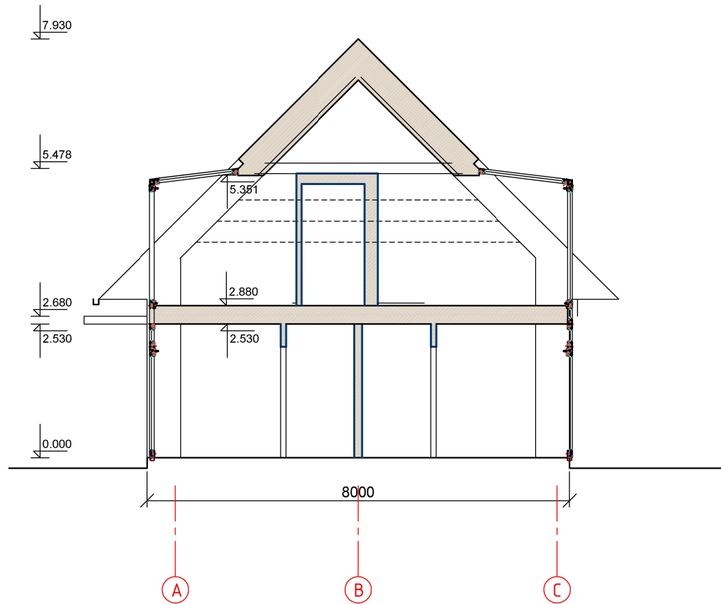
PJŪVIS 2 - 2 M 1:100
