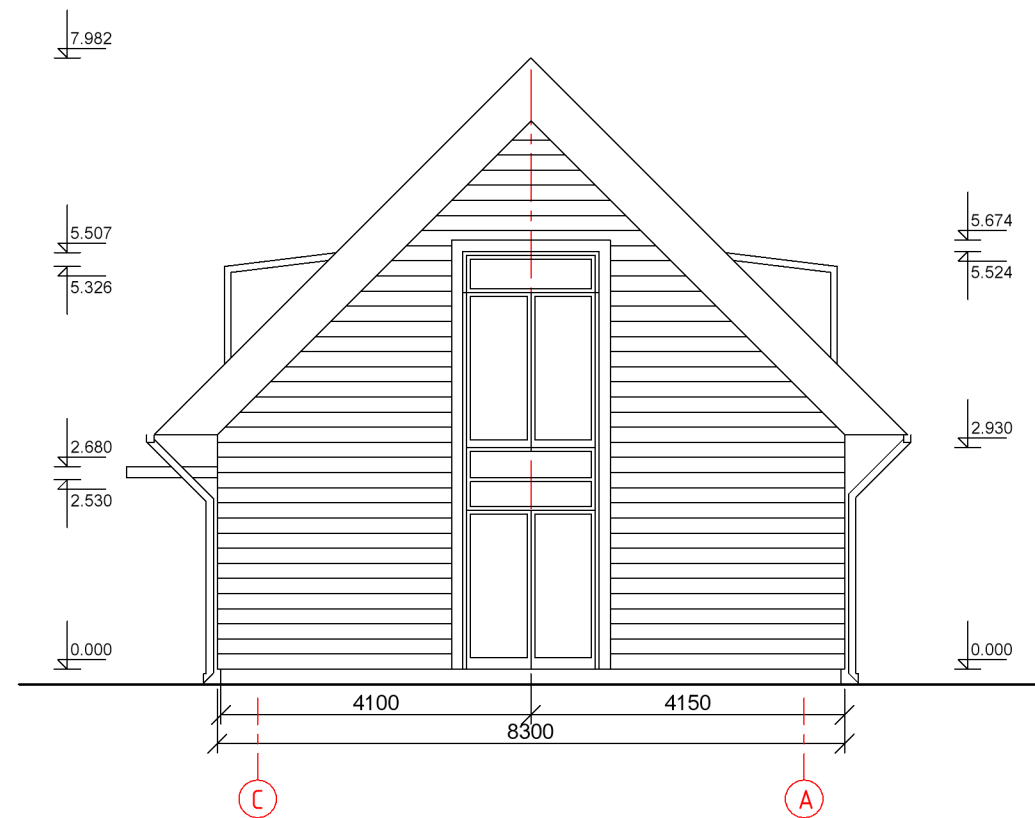
Fasadas C - A M 1:100
