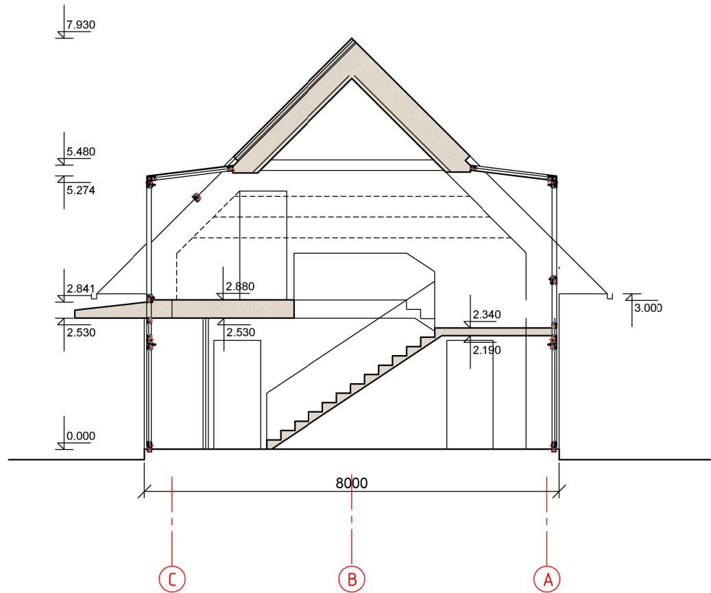
PJŪVIS 1 - 1 M 1:100
