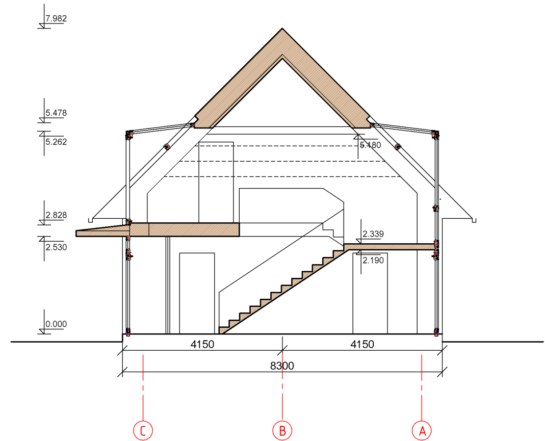
PJŪVIS 2 - 2 M 1:100
