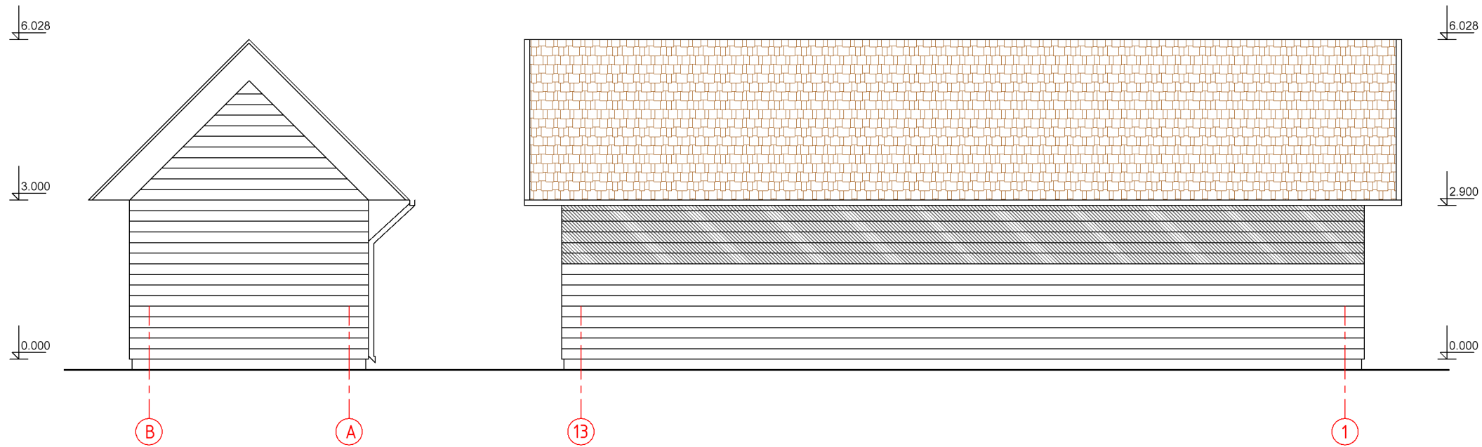
Fasadas B - A M 1:100
