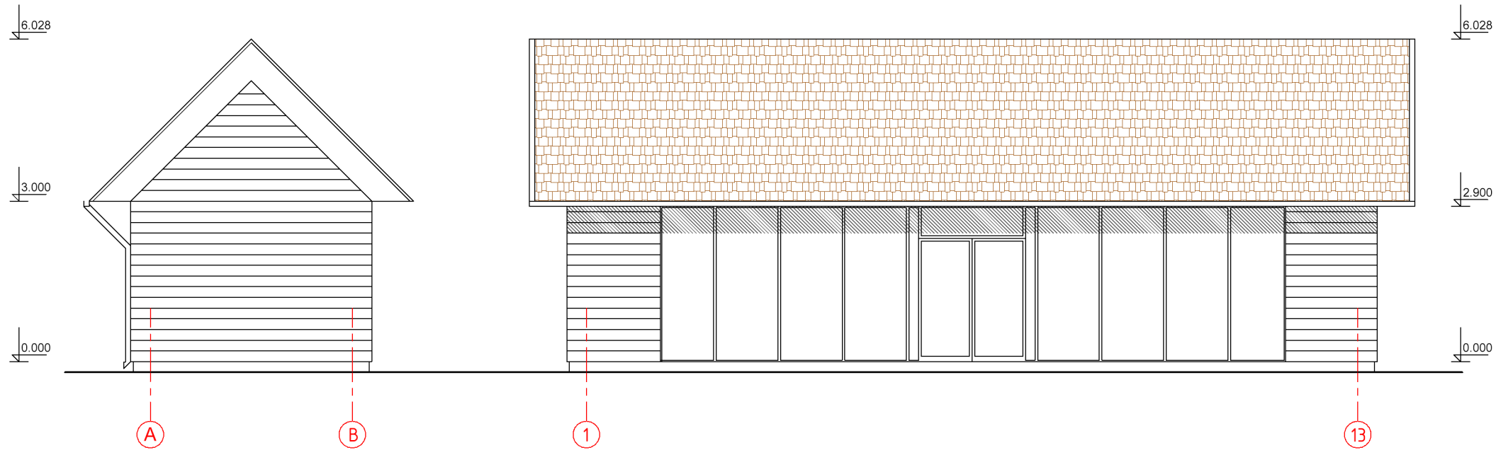
Fasadas A - B M 1:100
