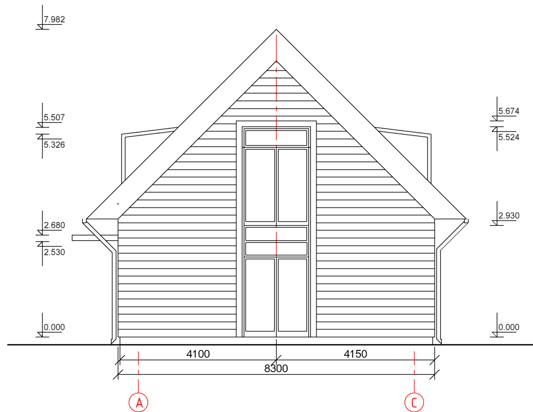
Fasadas A - C M 1:100
