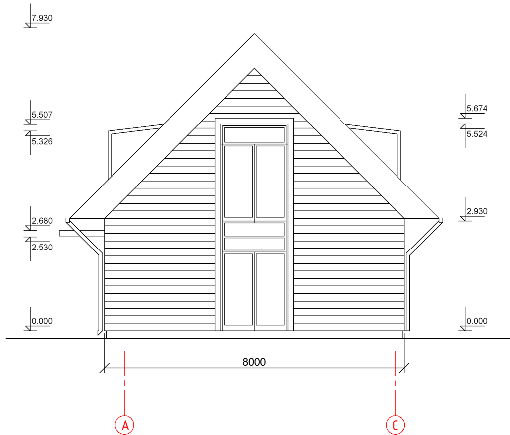
Fasadas A - C M 1:100
