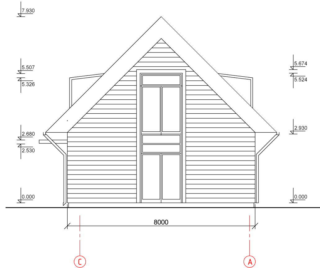
Fasadas C - A M 1:100
