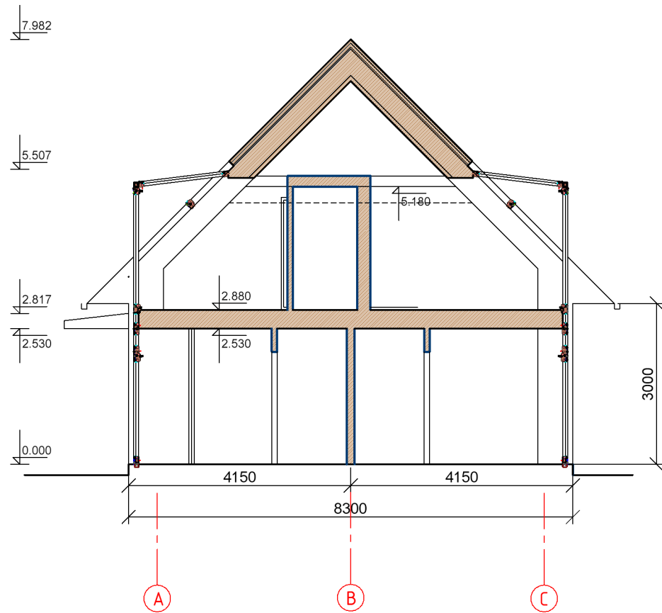
PJŪVIS 1 - 1 M 1:100
