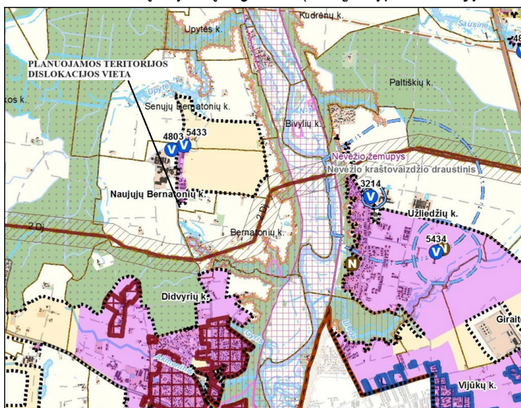
FRAGMENTAS IŠ KAUNO RAJONO SAVIVALDYBĖS GERIAMOJO VANDENS TIEKIMO IR NUOTEKŲ TVARKYMO INFRASTRUKTŪROS PLĖTROS SPECIALIOJO PLANO KEITIMO SPRENDINIŲ PAGRINDINIO BRĖŽINIO
